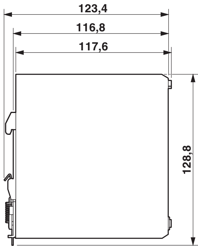
Desenho de medidas
