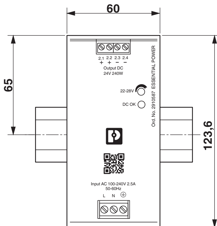
Desenho de medidas
